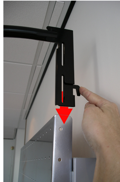
schuif haak in achterplaat
