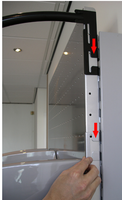
schuif haak in achterplaat
